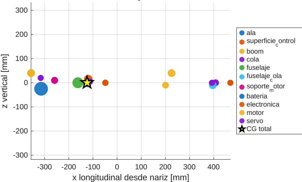
Distribucion de masa y CG - vista lateral
